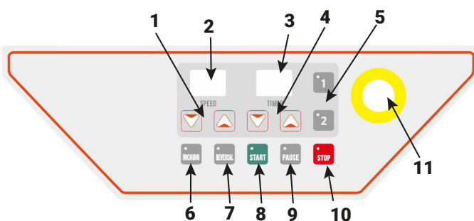
Abbildung 2 Bedienfeld
